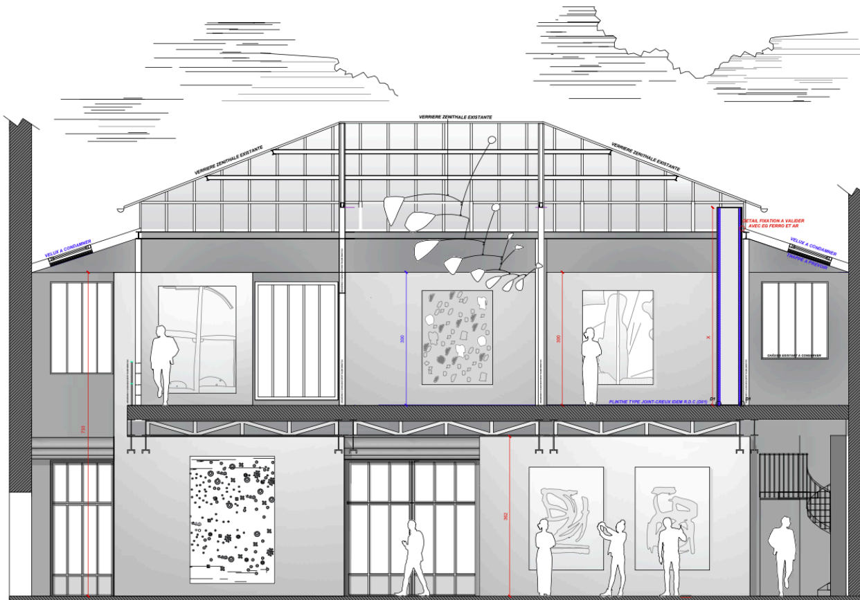
COUPE CC
