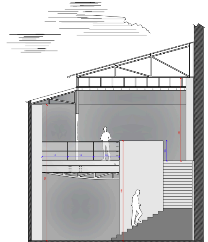
COUPE GG
